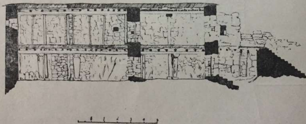
ბესო საბიევის სახლი სოფ. შავარდენში (მასშტაბი 1:50); სურ. 1. კრილი 1—1. სურ. 2. კრილი 2—2.
