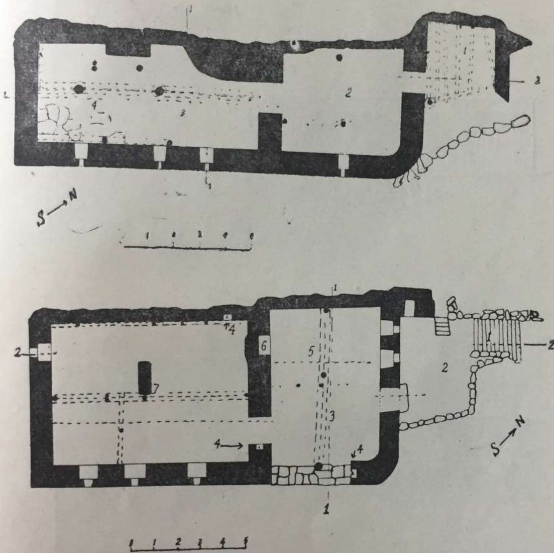
ბესო საბიევის სახლი სოფ. შავარდენში (მასშტაბი 1:50); სურ. 1. პირველი სართულის გეგმა: 1) საცხენე, 2) საბერწე, საძროხე 4) საცხვრე. სურ. 2. მეორე სართულის გეგმა: 1) კიბე, 2) საცხენის ბანი; 3) აივანი, 4) თახჩები, 5) სენე, 6) განჯინა, 7) სამყოფო.
