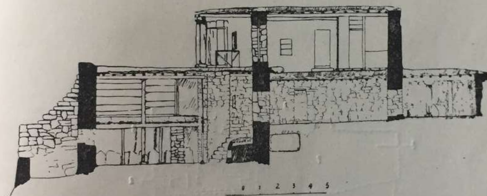
ივანე გუდიევის სახლი სოფელ ზემო ოქროყანაში (მასშტაბი 1:50); სურ. 1. გვერდითი ფასადი, სურ. 2. კრილი 2—2.
